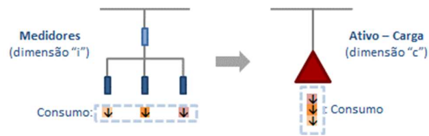
Figura 10: Exemplo de representação da agregação de dados de uma planta industrial com diversos pontos de medição associados. Destaca-se que a consolidação dos valores obtidos por ponto de medição em informações por ativo depende de um tratamento particular por meio de um conjunto de expressões específicas, conforme a configuração elétrica de cada instalação.
